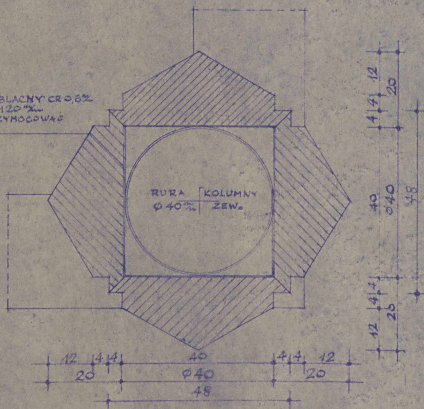
PRZĘKROJ POZIOMY DETALU „A” 1:1.
