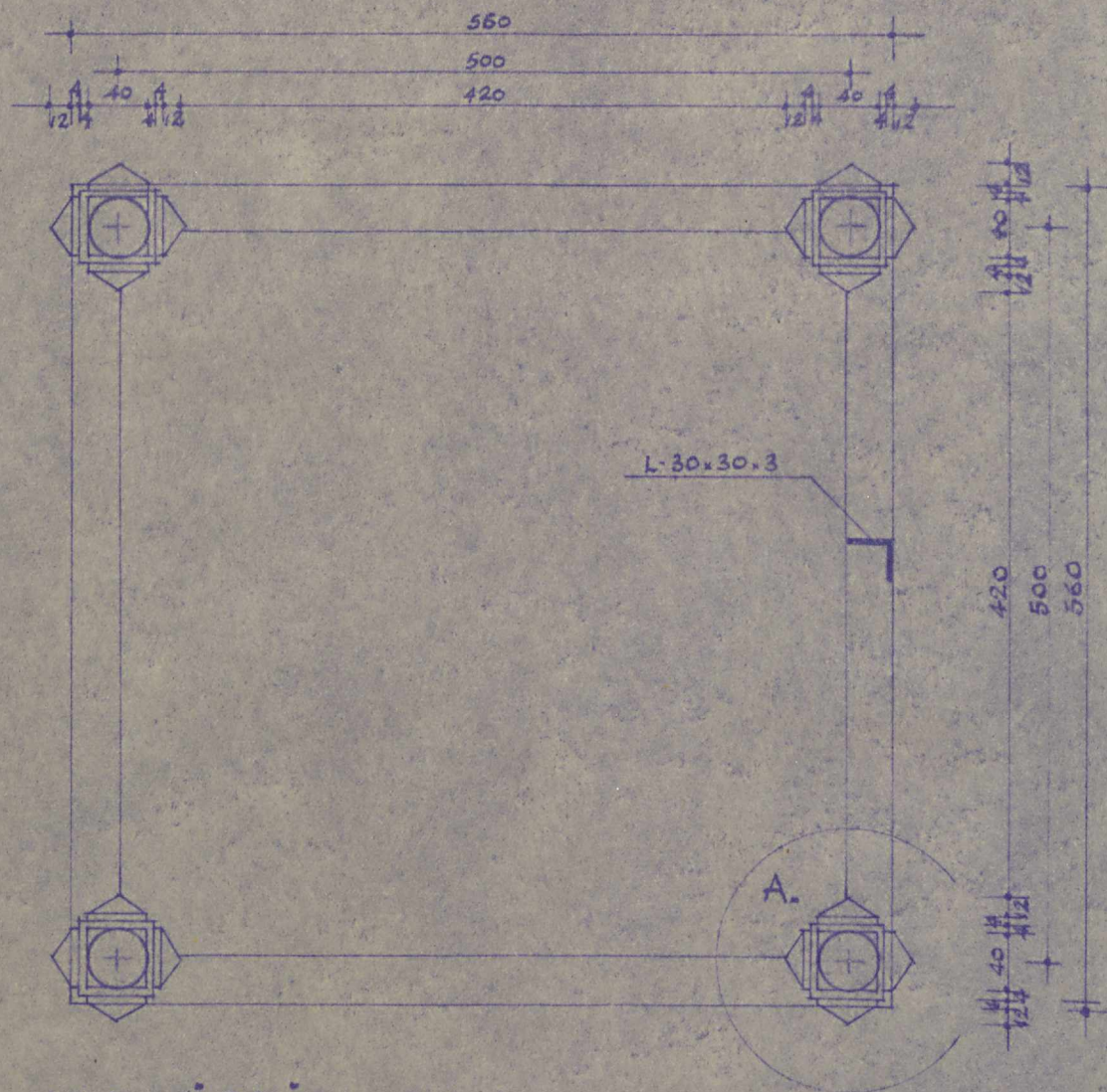
PRZĘKROJ POZIOMY-A-A. 1:5.
