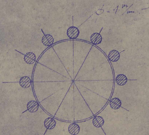
PRZEKROJ POZIOMY-DETAL-B.-1:1.
