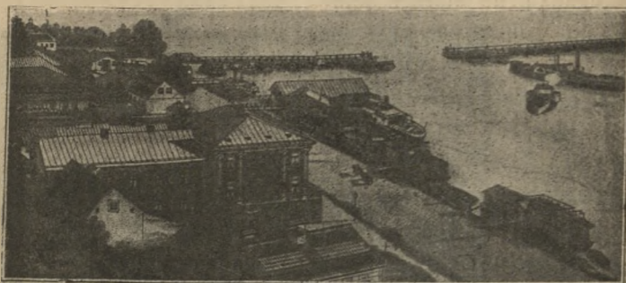
Most łyżwowy pod Płockiem, rozwiedziony w celu przepuszczenia statków parowych.
