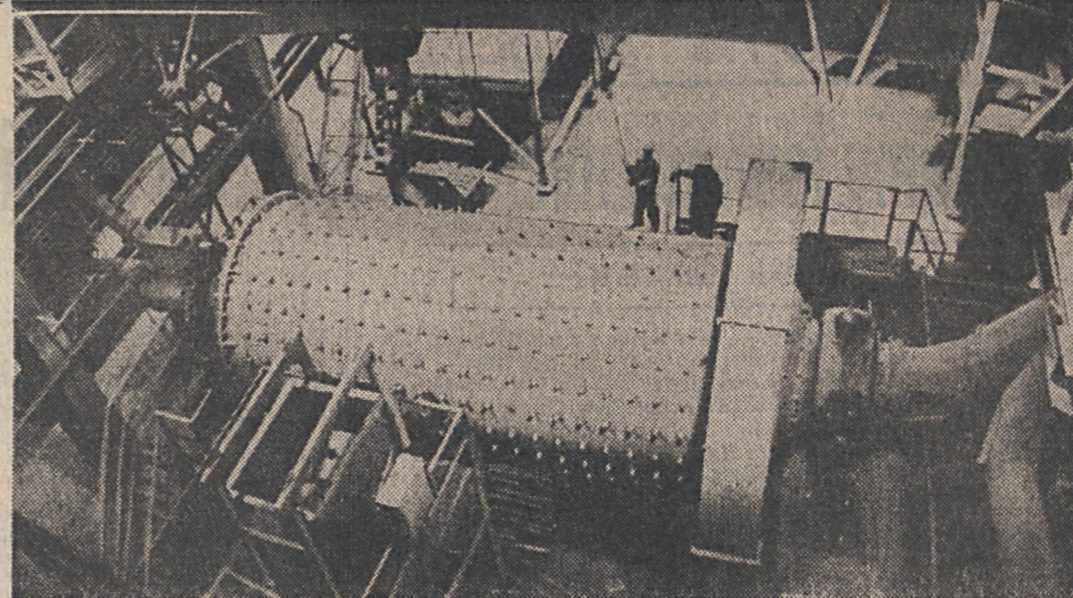
Mączka żużlowa jako nawóz W fabryce „Amurstał” w Komsomolsku pracują urządzenia do przemiału mączki żużlowej, która jest wykorzystywana w rolnictwie Dalekiego Wschodu do zwiększenia plonów. Fot. CAF — TASS
