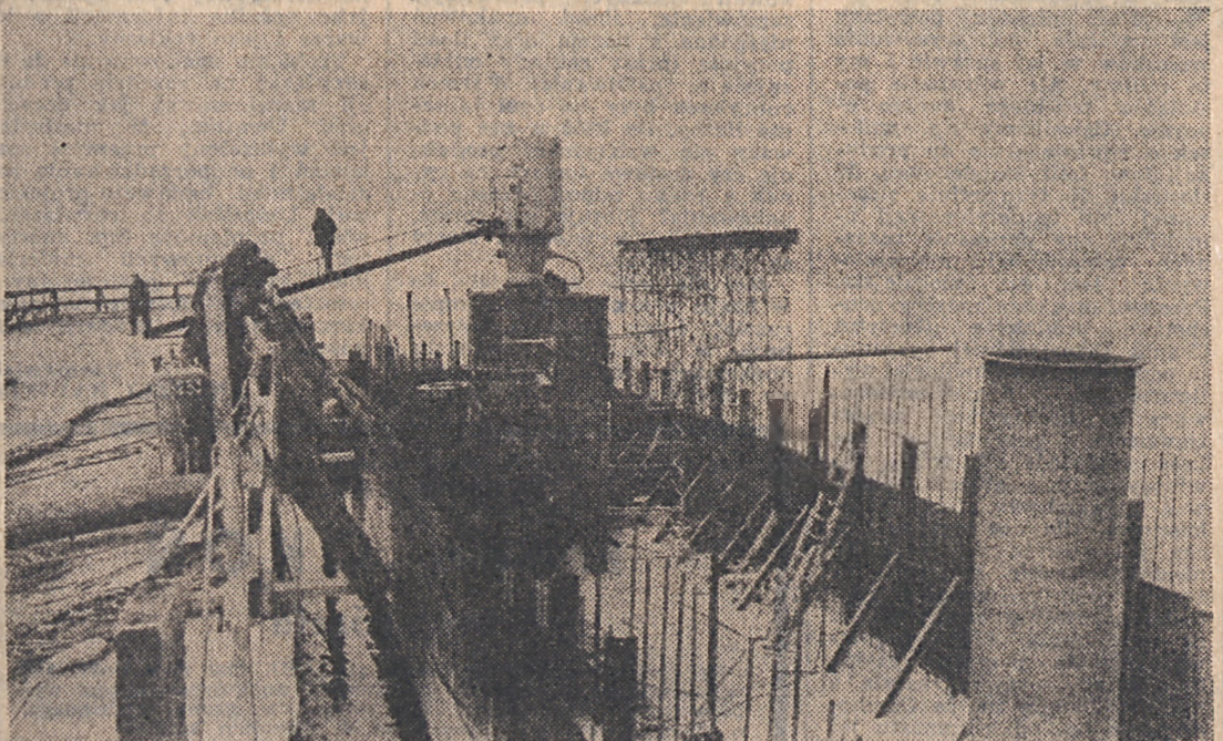
Budowa Mostu Tolstuskiego. Keson, który będzie podstawą jednej z podpór mostu osiadł na dnie Wisły. Teraz załoga PRK-15 przygotowuje się do wkopywania go w grunt i betonowania. Fot. Zdzisław Kwitka
