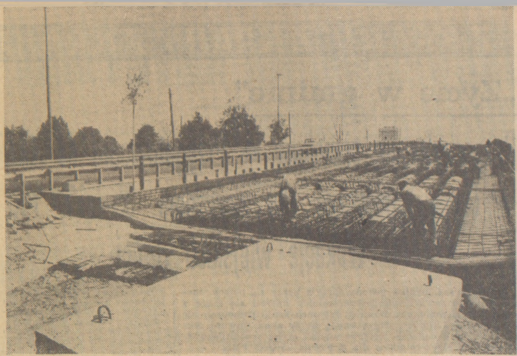
Trasa Modlińska. Za niespełna dwa miesiące Warszawa będzie miała nową arterię komunikacyjną. 9-kilometrowa trasa Modlińska nie tylko usprawni ruch w kierunku Zalewu Żegrzyńskiego, lecz także pełnić będzie funkcję trasy wylotowej w kierunku Gdańska. Na zdjęciu: pracownicy MPRI przygotowują do zabetonowania północny segment wiaduktu zachodniego przy skrzyżowaniu z ul. Płochocińską (w.m.) Fot. Zbigniew Furman
