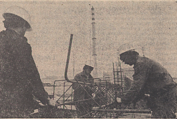
(A) Pomyślnie rozwija się polsko-francuska współpraca w przemyśle chemicznym. Jednym z jej przykładów jest rozbudowa kombinatu chemicznego „Police”. N/z: prace zbrojarskie przy fundamentach budynku głównego wytwórni nawozów trójskładnikowych.
