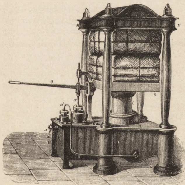
Prasa hydrauliczna.
