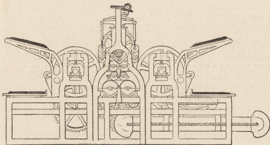
Pierwsza pospieszna maszyna drukarska.
