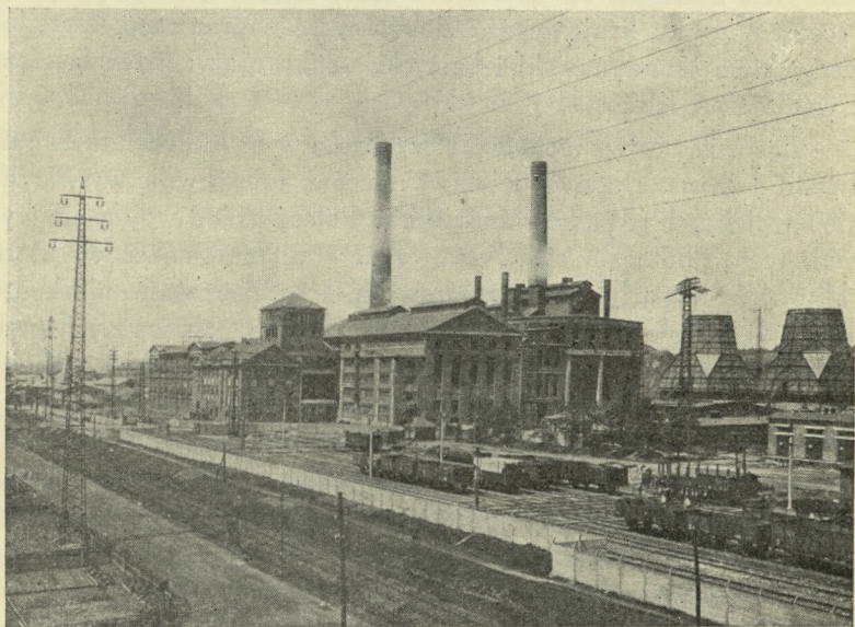
Śląskie Zakłady Elektryczne S. A. Katowice: Elektrownia w Łaziskach Górnych
