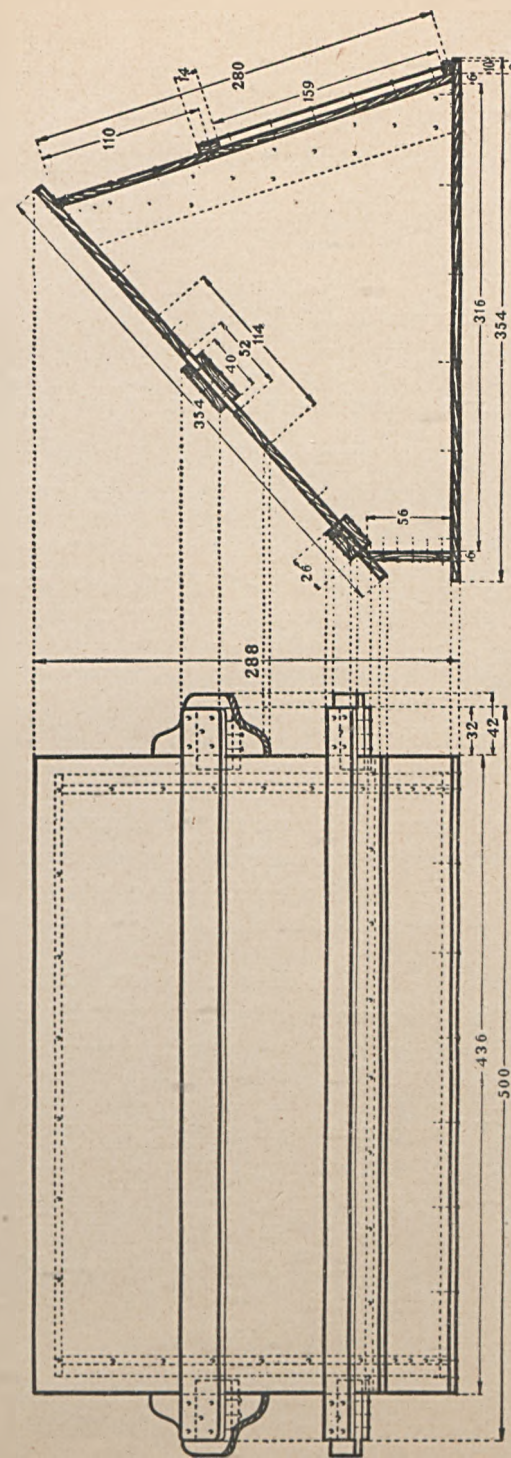
RYŚ. 18 c PULPIT DO PISANIA GRAFICZNEGO
