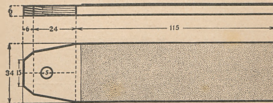
RYS. 7 a . DESECZKA DO OSTRZENIA OŁÓWKÓW
