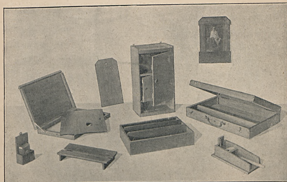
Modele na powtórzenie ćwiczeń: skrzyneczka wisząca na zapaliki, ławeczka do rozpinania motyli, paleta z pudełkiem do malowania, skrzyneczka na noże i widelce, pudełeczko na zapaliki i papierosy, skrzynka do farb, szafka wisząca, ramka, deseczka do krajania.
