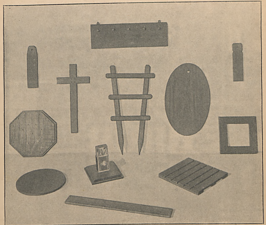
Modele: linijka (ćwicz. Nr. od 1 do 3 włącz.), wieszadełko (ćwicz. od 1 do 4 włącz.), podstawka do pudełka na zapalki (ćwicz. od 1 do 3 i od 5 do 7 włącz.), podstawka ośmiokątna (ćwicz. od 1 do 3 i od 5 do 8 włącz.), denko okrągłe (ćwicz. 9 i 10), deseczka elipsa (ćwicz. od 9 do 11), krzyż, drabinka do kwiatów (na powtórzenie ćwiczeń), etykieta (ćwicz. od 1 do 3 i 11, 12), deseczka do ostrzenia ołówków, podstawka listewkowa (na powtórzenie ćwiczeń), ramka kwadratowa (ćwicz. od 1 do 3 oraz 5 i 13).
