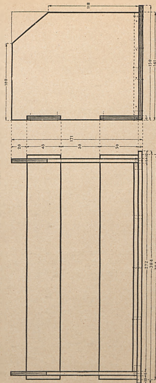
RYS. 14 c . PÓŁECZKA STOJĄCA DO KSIĄŻEK
