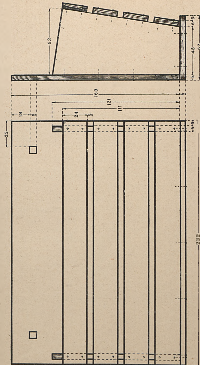
RYS. 13 b . PUDEŁKO WISZĄCE NA LISTY
