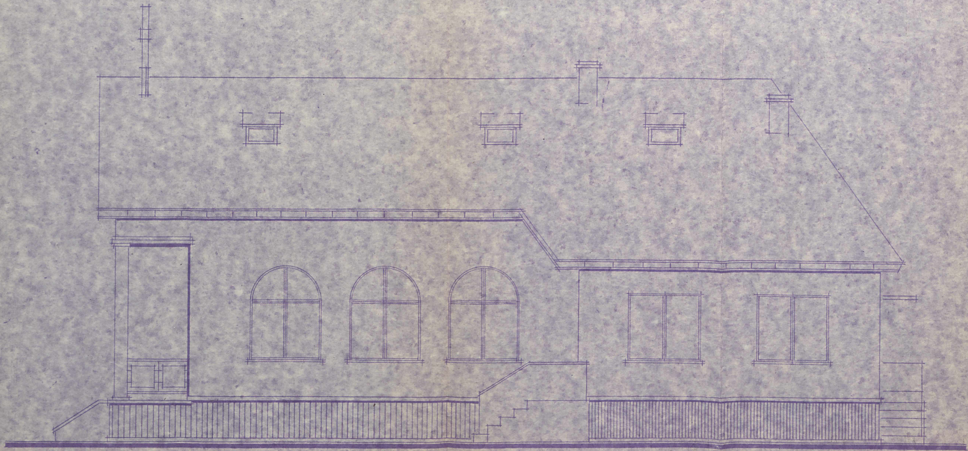
ELEKASTA ZACHODNIA 1-50
