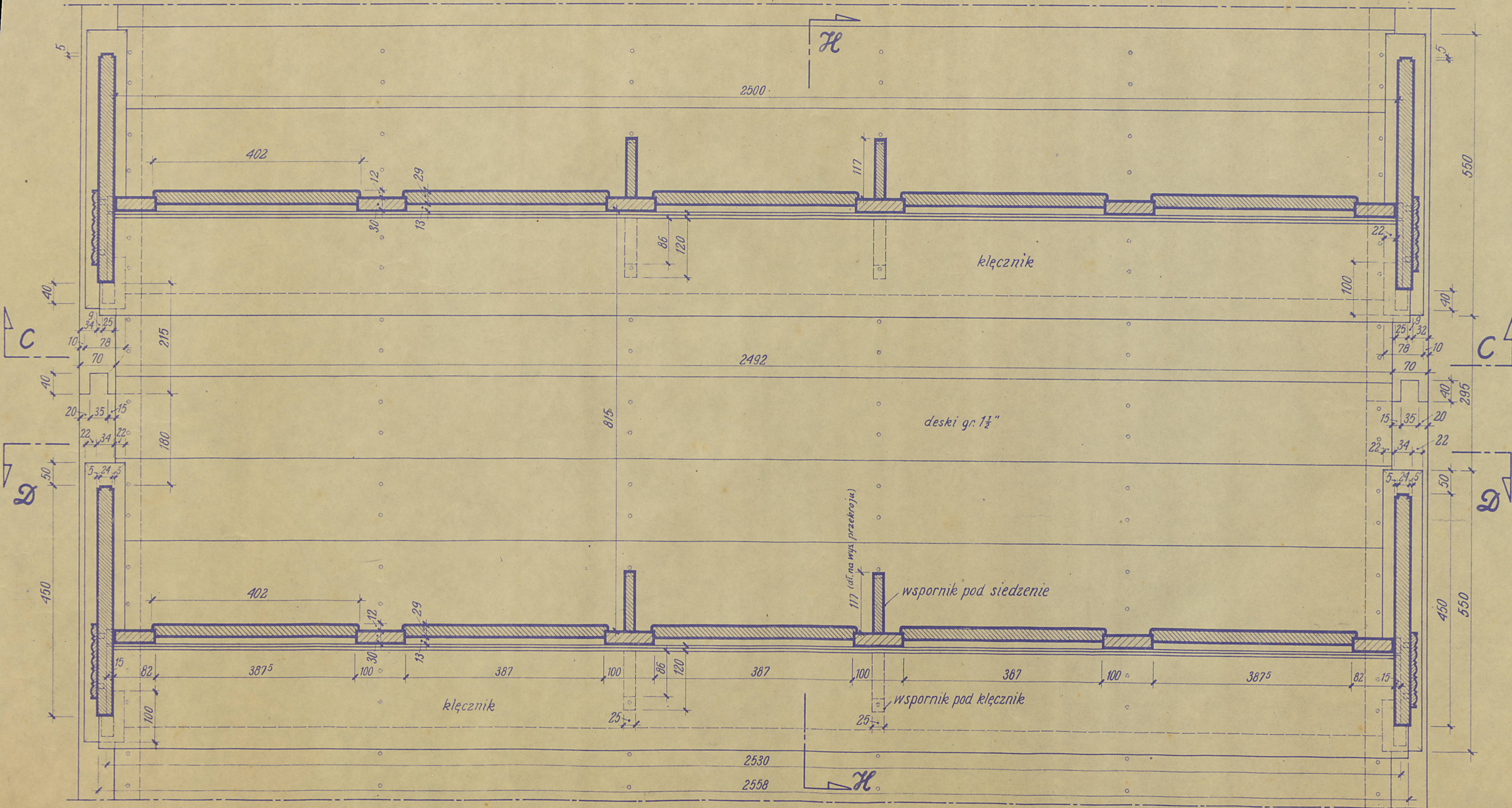
Projekt ławek - Rzut na wys. przekroju A-A skala 1:5 (część środkowa)
